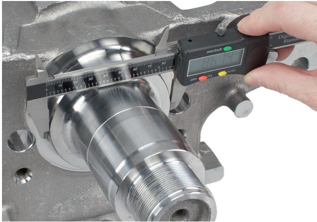
Şekil 2: Üç koruyucu halkadan hangisinin monte edilmesi gerektiğini belirlemek için, sızdırmazlık elemanı yuvasının çapı ölçülmelidir.
