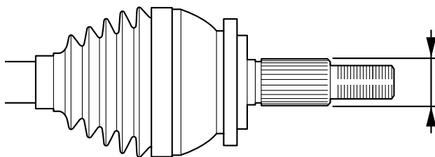
Рисунок 1: Чтобы идентифицировать правильный подшипник, необходимо измерить внешний диаметр шлицевой секции вала ШРУСа
