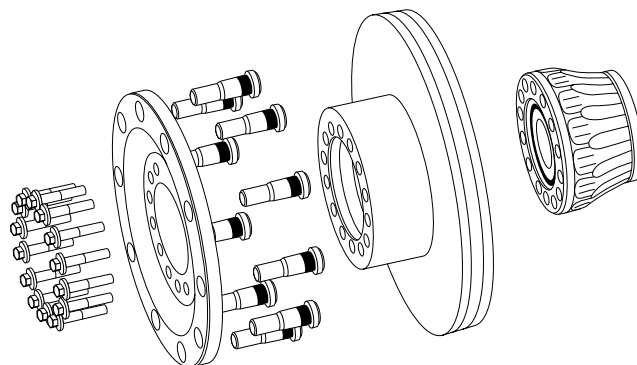
Зображення 1: Для вісей з номером S63U, крім модуля колісного підшипника, необхідно також замінити гальмівний диск, кріплення колеса, шпильки для кріплення колеса і гайки
