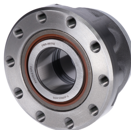
Afbeelding 1: Het onderdeel nr. 805532.01.H195 is voorzien van een afdichting.
