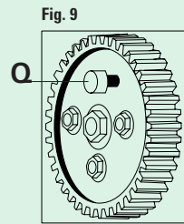
FIGURA 9 Inserire l'apposito attrezzo di bloccaggio della puleggia della pompa di iniezione Q.
