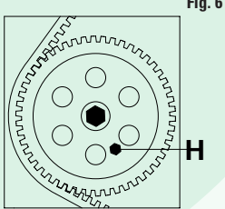
FIGURA 6 Inserire l'apposito attrezzo di bloccaggio della puleggia della pompa di iniezione H.
