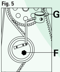
FIGURA 5 Allentare il bullone di bloccaggio F ed inserire l'apposito attrezzo di tensionamento con il relativo peso G 120 mm; verificare che il braccio dell'attrezzo rimanga in posizione orizzontale e serrare, quindi, il bullone di bloccaggio F.
