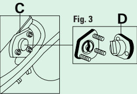
FIGURA 1 Controllare il corretto allineamento delle tacche di fase A (per motori non turbo). FIGURA 2 Controllare il corretto allineamento delle tacche di fase B (per motori turbo) FIGURA 3 Togliere il depressore dal lato posteriore della testata C ed inserire l'apposito attrezzo di bloccaggio dell'albero a camme D. FIGURA 4 Inserire l'apposito attrezzo di mantenimento della tensione sulla puleggia dell'albero a camme E.
