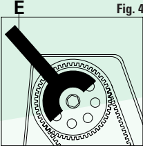
FIGURA 1 Controllare il corretto allineamento delle tacche di fase A (per motori non turbo). FIGURA 2 Controllare il corretto allineamento delle tacche di fase B (per motori turbo) FIGURA 3 Togliere il depressore dal lato posteriore della testata C ed inserire l'apposito attrezzo di bloccaggio dell'albero a camme D. FIGURA 4 Inserire l'apposito attrezzo di mantenimento della tensione sulla puleggia dell'albero a camme E.
