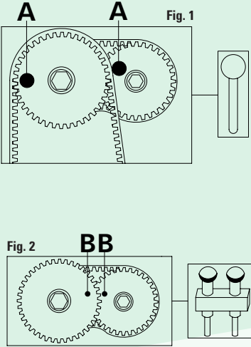
FIGURA 1 Inserire gli appositi attrezzi di bloccaggio degli alberi a camme A. FIGURA 2 Inserire l'apposito attrezzo di bloccaggio degli alberi a camme B.
