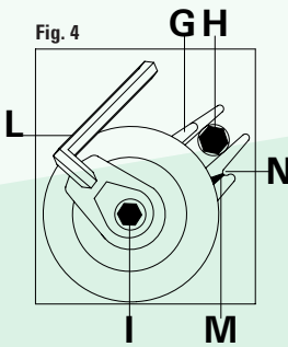
FIGURA 4 Assicurarsi che la piastra G sia fissata al di sotto del bullone di bloccaggio H; allentare il bullone di blocco I e ruotare in senso orario il tendicinghia utilizzando la chiave L sull'eccentrico di registro; allineare l'indicatore M con la tacca N e serrare, quindi, il bullone di bloccaggio I.
