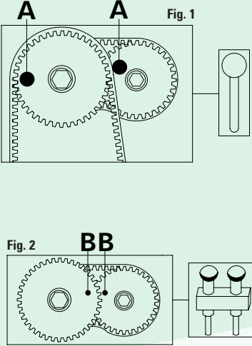
FIGURA 1 Insertar la herramienta especial de inmovilización de árbol de levas A. FIGURA 2 Insertar la herramienta especial de inmovilización de árbol de levas B.
