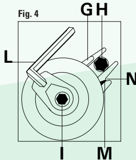
FIGURA 4 Asegurarse que la lamina C esta fijada por debajo del tornillo de fijación H. Luego aflojar el tornillo de fijación I, y girar el tensor de la correa en sentido de las agujas del reloj actuando con la llave L sobre el excéntrico de regulación hasta lograr la alineación de la marca M con la muesca N. Por último, apretar el tornillo de fijación I.
