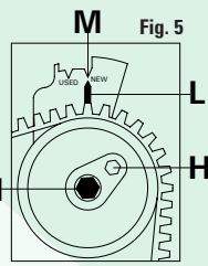
FIGURA 4 Aflojar el tornillo de fijación D. Girar el tensor de la correa sobre el excéntrico de regulación E, en sentido de las agujas del reloj hasta lograr que el indicador F quede alineado con la muesca de fase G. Por último, apretar el tornillo de fijación D. FIGURA 5 Aflojar el tornillo de fijación L. Girar el tensor de la correa sobre el excéntrico de regulación H en sentido de las agujas del reloj. Luego, alinear el indicador L con la muesca de fase M. Por último apretar el tornillo de fijación L.
