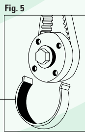
FIGURA 4 Insertar la herramienta de inmovilización del volante motor F. FIGURA 5 Insertar la herramienta especial de inmovilización de correa de distribución G.
