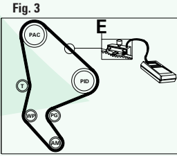
FIGURA 2 Aflojar el tornillo de fijación C. Girar el tensor de la correa en sentido contrario a las agujas del reloj utilizando para ello la herramienta tensora insertada en D hasta obtener la medida correcta de tensión. Apretar el tornillo de fijación C. FIGURA 3 Insertar la herramienta apropiada para medición de la tensión de correa E en el punto indicado, y actuar sobre el tensor de la correa hasta conseguir un valor de tensión de 51 ± 3 unidades SEEM.
