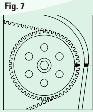
FIGURA 7 Verificar la correcta alineación de las marcas de puesta en fase H (Bomba Bosch). FIGURA 8 Verificar la correcta alineación de la marca de puesta a punto I (Bomba Lucas).
