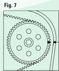
FIGURA 7 Controllare il corretto allineamento delle tacche di fase H (pompa Bosch). FIGURA 8 Controllare il corretto allineamento della tacca di fase I (pompa Lucas).
