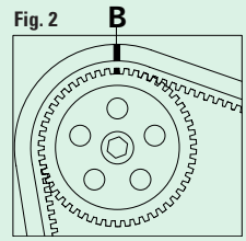
FIGURA 1 Verificar que la marca de puesta a tiempo este en línea con la marca del cárter de la distribución A. FIGURA 2 Verificar la correcta alineación de las marcas de puesta en fase B.
