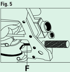
FIGURA 5 Insertar la herramienta especial para inmovilización de cigüeñal motor F. FIGURA 6 Verificar la correcta alineación de las marcas de puesta en fase G.
