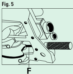
FIGURA 5 Inserire l'apposito attrezzo di bloccaggio dell'albero motore F. FIGURA 6 Controllare il corretto allineamento delle tacche di fase G.
