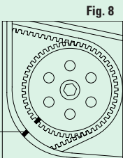
FIGURA 7 Verificar la correcta alineación de las marcas de puesta en fase H (Bomba Bosch). FIGURA 8 Verificar la correcta alineación de la marca de puesta a punto I (Bomba Lucas).
