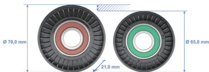
画像 2：ガソリンエンジン車向け偏向プーリー 532 0404 30 (左) とディーゼルエンジン車向け偏向プーリー 532 0406 30 (右)
