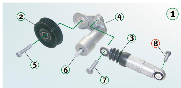
Obrázek 1: Detailní znázornění 534 0014 10 se všemi komponenty
