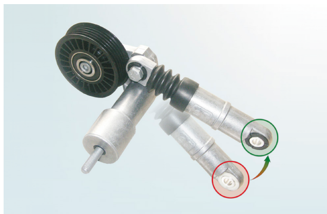
Obrázek 2: 534 0014 10 – provedení s bílými a černými plastovými pouzdry upevňovacích ok hydraulického tlumiče
