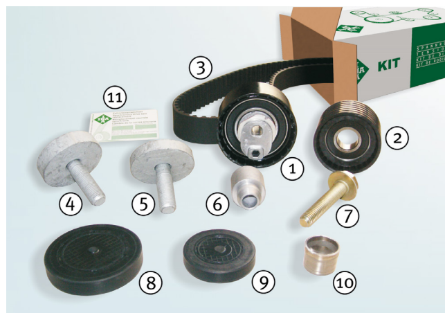
Bilder 1: registerremsett 530 0363 10
