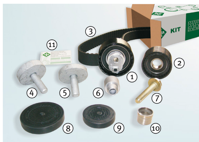
Рисунок 1: Комплект ремня ГРМ 530 0363 10
