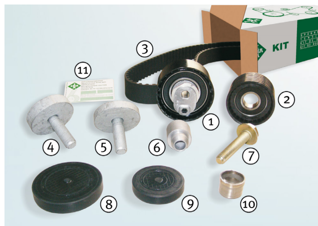
Bild 1: komplett innehåll i kuggremsatsen - INA KIT 530 0363 10
