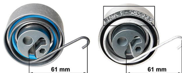
Obrázek 1: 531 0535 20 - Vlevo je staré provedení, vpravo je nové provedení
