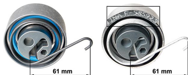
Рисунок 1: 531 0535 20 - прежняя конструкция (слева), новая конструкция (справа)
