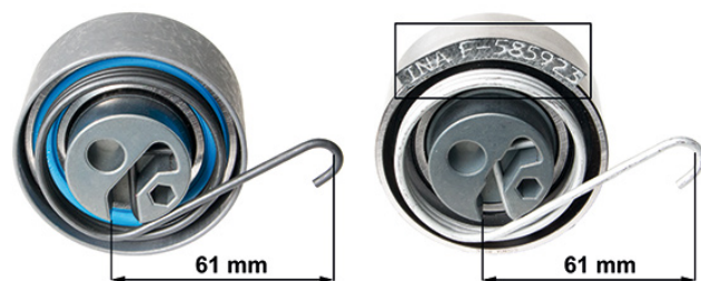
Bild 1: 531 0535 20 - till vänster hittillsvarande utförande, till höger nytt utförande
