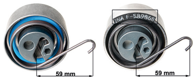
Bild 2: 531 0819 10 - till vänster hittillsvarande utförande, till höger nytt utförande
