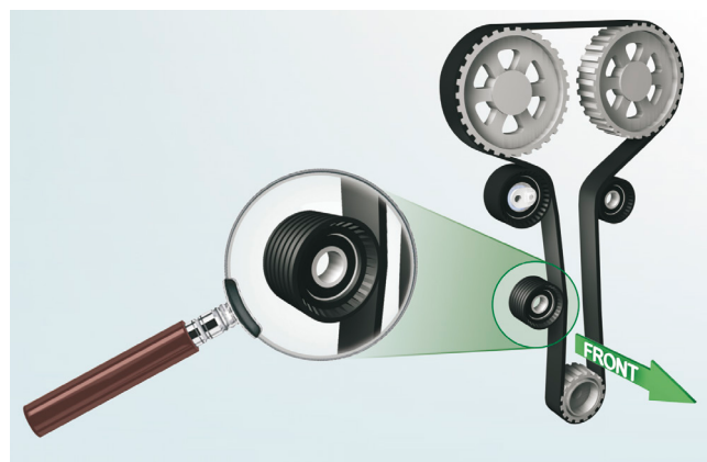
Снимка 1: Път на ремъка и позиции на ролката в двигател F4R
