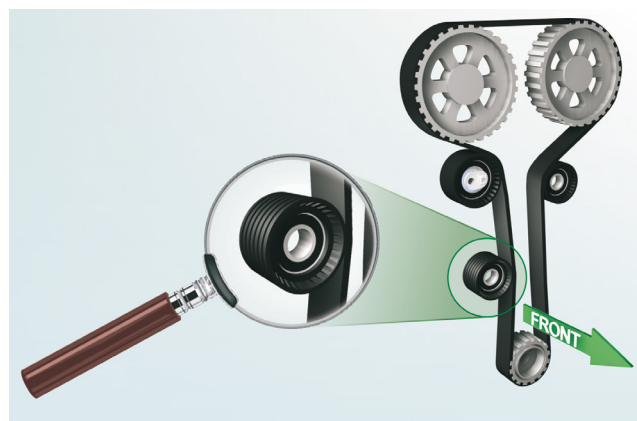
Bild 1: Remföring och läge hos rullar i motor F4R
