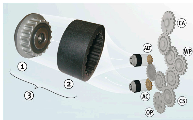
Εικόνα 1: Ελεύθερη περιστροφή γεννήτριας με εύκαμπτο σύνδεσμο και μετάδοση κίνησης με γρανάζια
