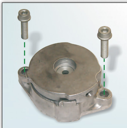
Obrázok 1: INA – vyhotovenie so dvomi skrutkami M8x35
