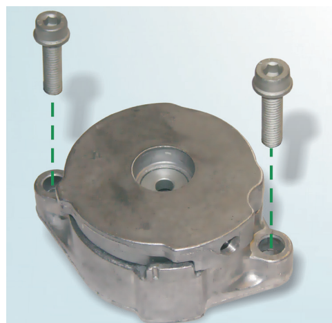
Зображення 1: Версія INA з двома гвинтами M8x35
