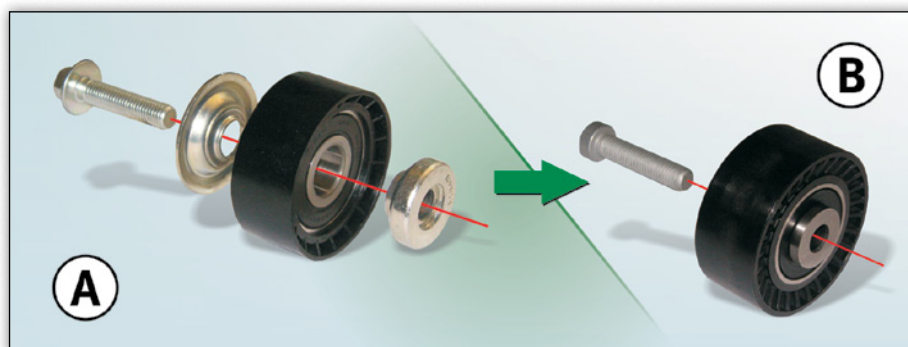
Polea de inversión 532 0433 10, versión anterior (A) y versión nueva (B)
