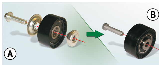
Kuva 1: Ohjainrulla 532 0433 10. (A) Edellinen malli. (B) Uusi malli
