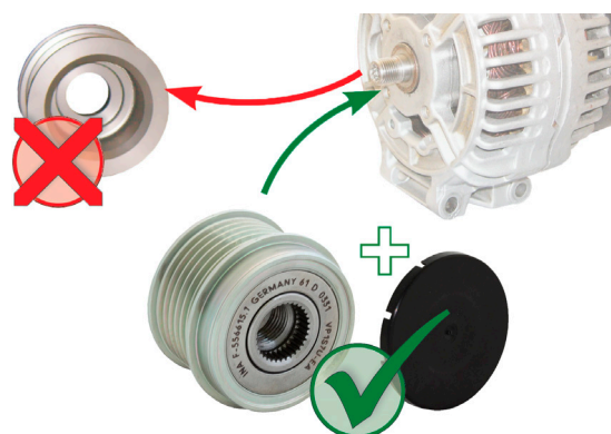
Рисунок 1: Замена цельного шкива на шкив генератора с обгонной муфтой
