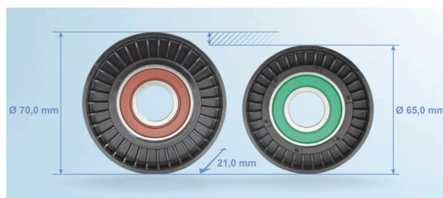
Figura 2: Fulia defletoare 532 0404 30 pentru vehiculele cu motor pe benzină (stânga) și fulia defletoare 532 0406 30 pentru vehiculele cu motor diesel (pe motorină) (dreapta)
