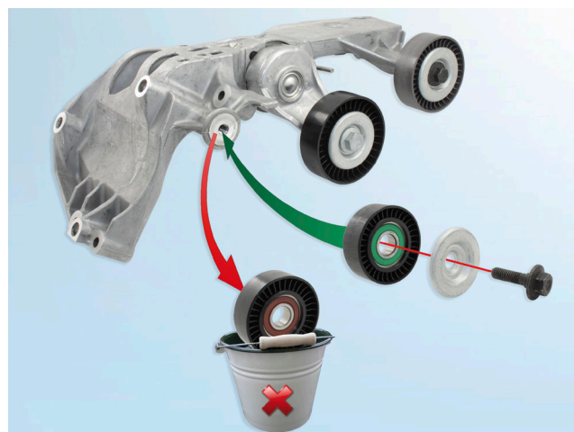
Figura 1: Unitate întinzătoare 534 0243 10
