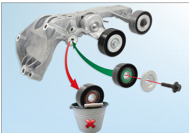
Slika 1: 534 0243 10 napenjalna naprava
