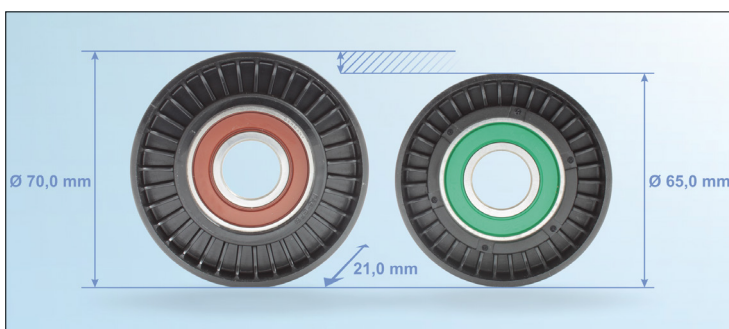
Slika 2: Preusmerjevalni valj 532 0404 30 za vozila z bencinskim motorjem (na levi) in preusmerjevalni valj 532 0406 30 za vozila z dizelskim motorjem (na desni)
