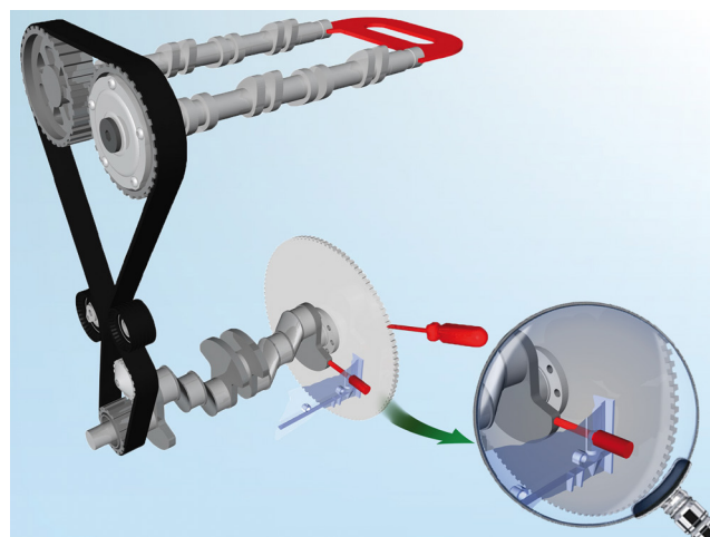
Figur 1: Registerremdrev med låseplate til kamskål (rød) på plass, innstillingspinne til kamskål (rød) og låseverktøy til svinghjul (rød)
