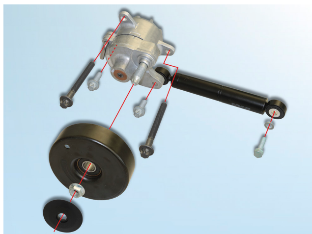
Obrázek 1: 533 0116 10 – oprávérenská sada INA pro pohon agregátů včetně upevňovacích šroubů
