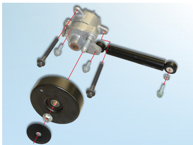
Kuva 1: 533 0116 10 – apulaitekäyttöjen INA-korjaussarja kiinnitysruuveineen
