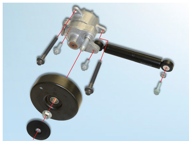
Зображення 1: 533 0116 10 - Ремонтний комплект натяжних роликів приводу допоміжних механізмів INA з гвинтами для кріплення
