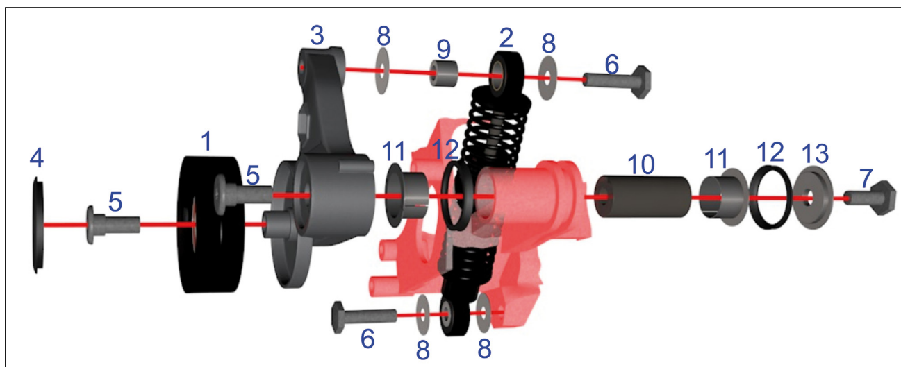
Slika 3: 533 0118 10 — garnitura za popravilo napenjalne naprave INA
