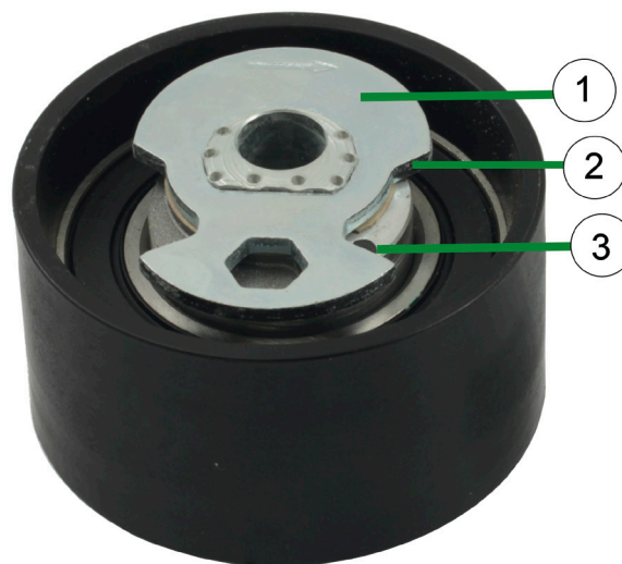
Obrázek 1: 531 0504 10 – poloautomatická napínací kladka
