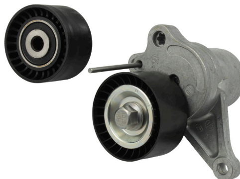
Рисунок 2: Пластиковый натяжной ролик и обводной ролик.
