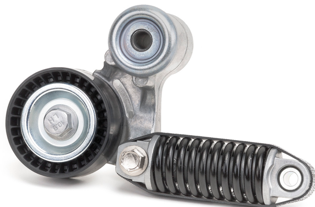
Снимка 1: 534 0314 10- обтегач за многоканални ремъци
