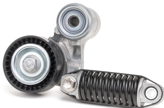
Kuva 1: 534 0314 10 – hihnan kiristin moniurakiilahihnaa varten
