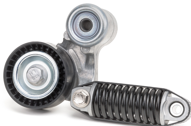
Bild 1: 534 0314 10 - spännare till multiribbrem
