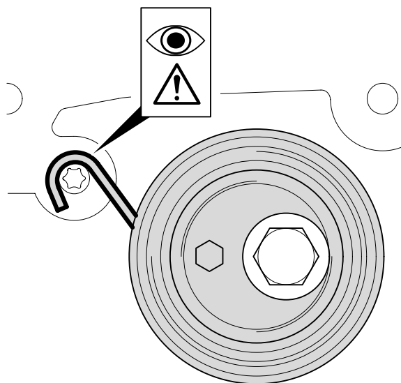
Kuva 1: Jousen oikea asennusasento lukitustapissa
