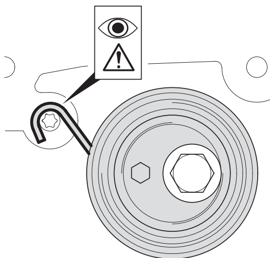
Afbeelding 1: Correcte inbouwpositie van de veer op de borgbout
