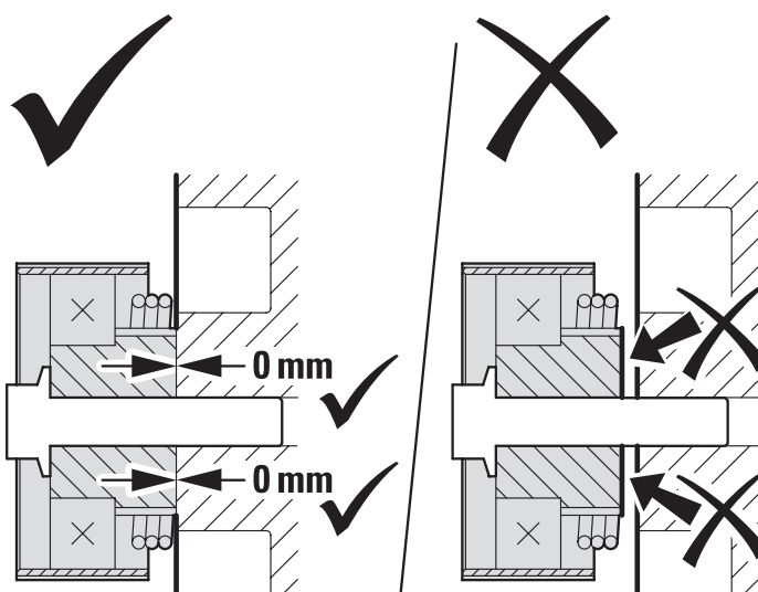
Afbeelding 2: Links – spanrol is over het volledige oppervlak op het opschroefvlak van de motor gemonteerd Rechts – spanrol is niet over het volledige oppervlak op het opschroefvlak van de motor gemonteerd
