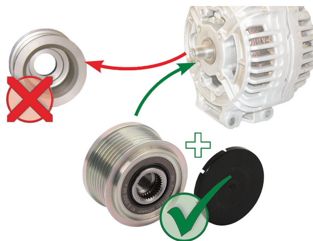
Cambio de polia rígida a uma polia livre de alternador
