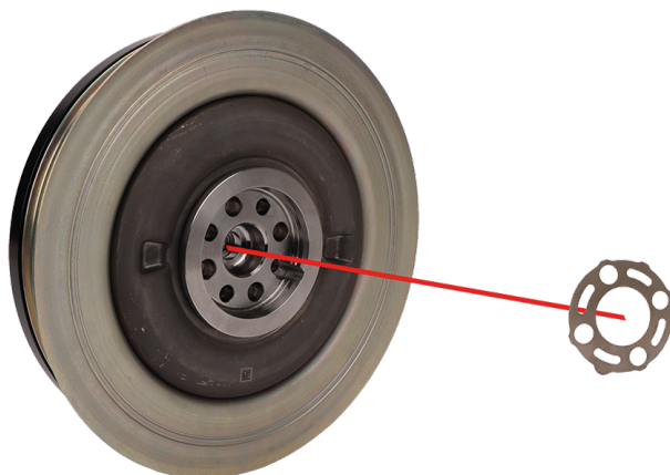
Obrázek 1: Řemenice FEAD na straně klikové hřídele s diamanty potaženou podložkou. U výše uvedených sad je tato podložka již vložena v montážní poloze na řemenici
