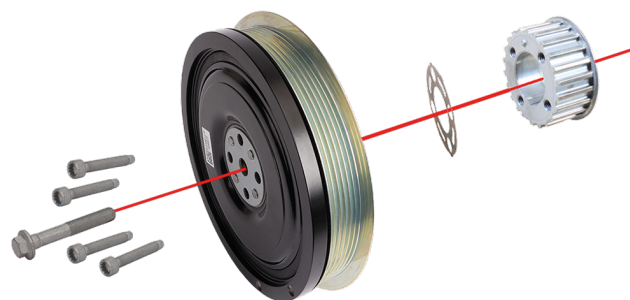
Obrázek 2: Šrouby řemenice, centrální šroub klikové hřídele, řemenice s tlumičem vibrací a diamanty potažená podložka
