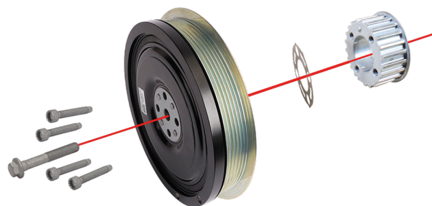
Figura 2: Șuruburi ale decuplorului fuliei de curea, șurub central al arborelui cotit, decuplor al fuliei de curea și șaibă diamantată
