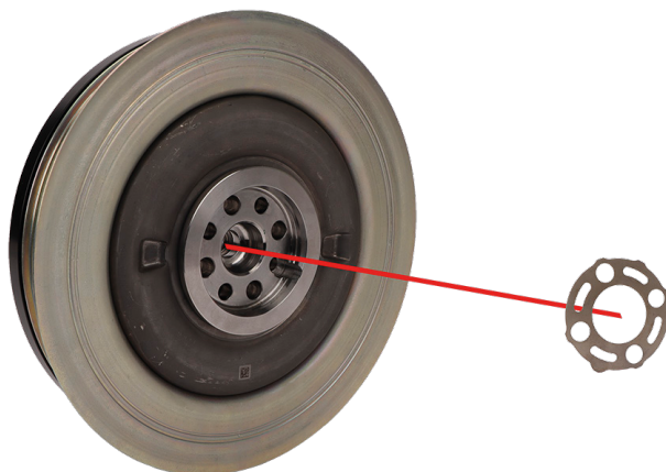
Figura 1: Partea dinspre arborele cotit a decuplorului fuliei de curea cu șaiba diamantată. În KIT-urile menționate mai sus, șaiba diamantată este deja introdusă în poziția de montare pe decuplorul fuliei de curea.
