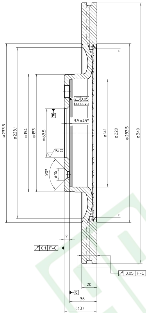
Sezione D-D
