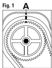
FIGURA 1 Verificar la correcta alineación de las marcas de puesta en fase A.
