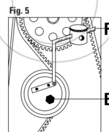
FIGURA 5. Aflojar el tornillo de fijación E, e insertar la herramienta especial de tensado de correa con su relativo peso F (65mm o 70mm); verificar que el brazo de la herramienta se mantenga en posición horizontal; Por último, apretar el tornillo de fijación E.
