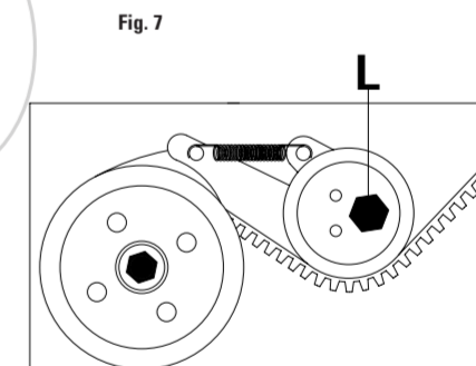
FIGURA 7 Allentare il bullone di bloccaggio L del tenditore della pompa di iniezione diesel; ruotare l'albero motore di 1/2 giri e serrare, quindi, il bullone di bloccaggio L.
