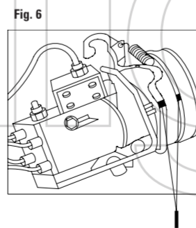
FIGURA 6 Controllare il corretto allineamento delle tacche di fase I.
