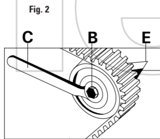
FIGURA 2 Allentare il bullone di bloccaggio B e ruotare in senso orario il tendicinghia utilizzando la chiave C, fino ad allineare il bordo destro dell'indicatore D del tendicinghia, con il bordo destro dell'indicatore E; serrare, quindi, il bullone di bloccaggio B.
