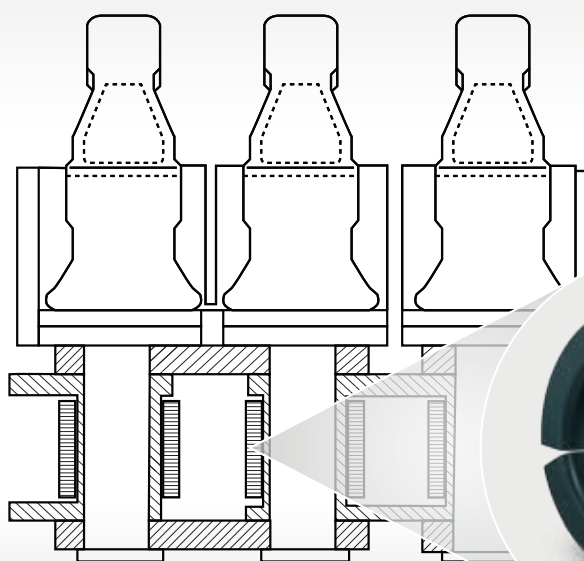
Ułożyskowanie macek z tulejami kołnierzowymi PERMAGLIDE® P10
