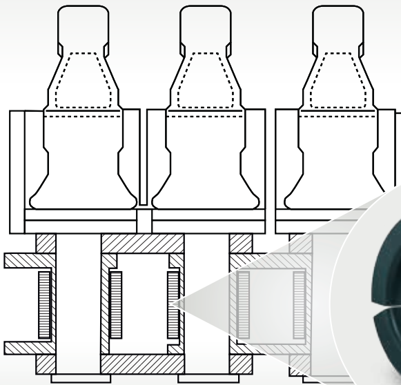
KS PERMAGLIDE® P10 kaymalı yataklı flanşlı gömlekler ile kısıkaç yataklaması
